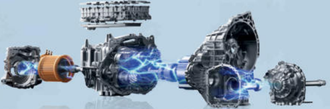
Transmisión longitudinal 2DHT
